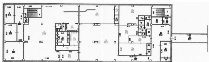
ПОЭТАЖНЫЙ ПЛАН ПОМЕЩЕНИЙ 4-ГО ЭТАЖА
