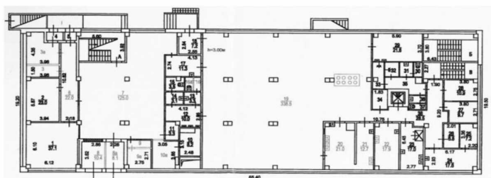
ПОЭТАЖНЫЙ ПЛАН ПОМЕЩЕНИЙ 3-ГО ЭТАЖА
